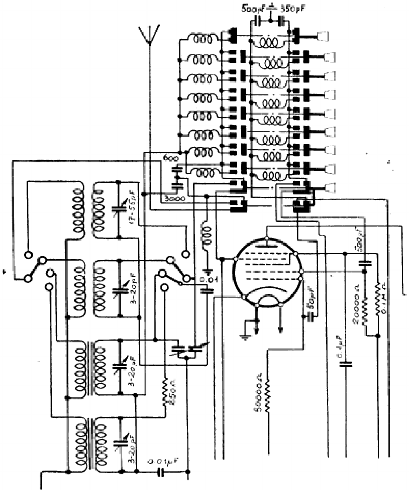
36. — Variazione per il C. G. E. Mod. 741 B. (Corrisponde al mod. 741 della pagina precedente, salvo per la variante).
